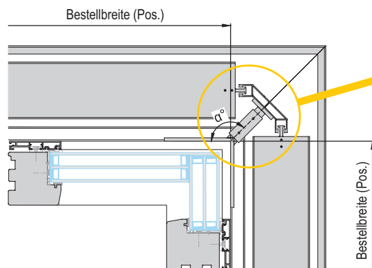
rohová vodící lišta
