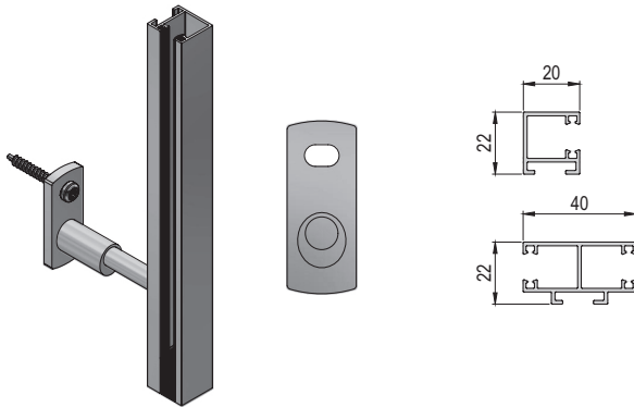
vodící lišty RAFA s teleskopickým držákem
